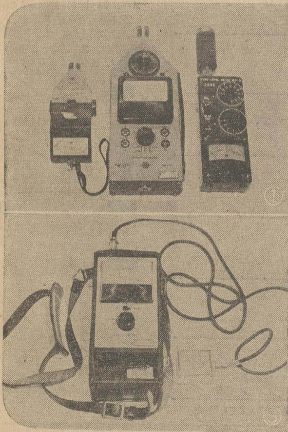
①●騒音を測定する指示騒音計、精密騒音計 ②●周波数分析機、レベルコーダー ③●振動のタテヨコ波を地表面で計る振動計
